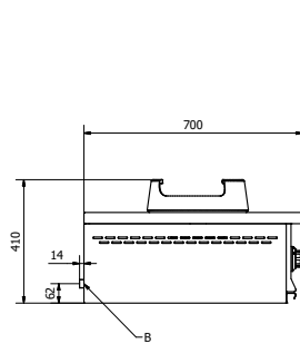
OPCIÓN QUEMADOR WOK 18kw WOK BURNER GAS CIRCUIT 18kw
